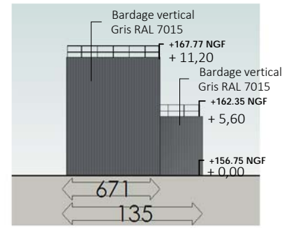
3 Façade Est 1 : 500
