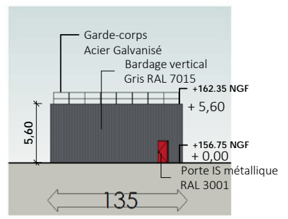
5 Façade Ouest 1 : 500
