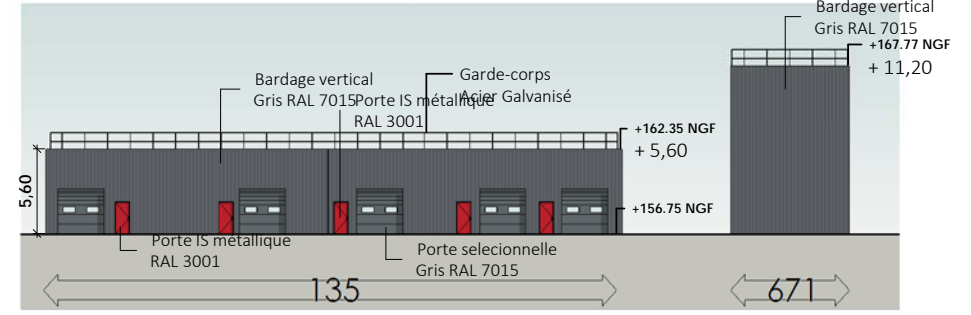
6 Façade Sud 1 : 500
