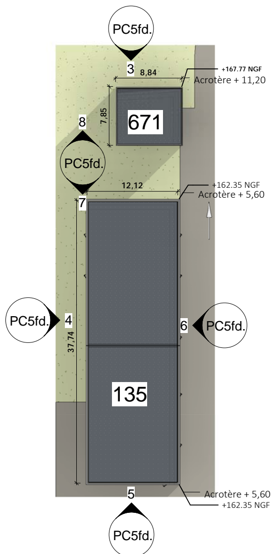
1 Plan de Toiture 1 : 500
