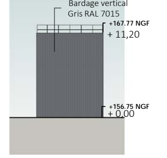
8 Façade Est -B671 1 : 500
