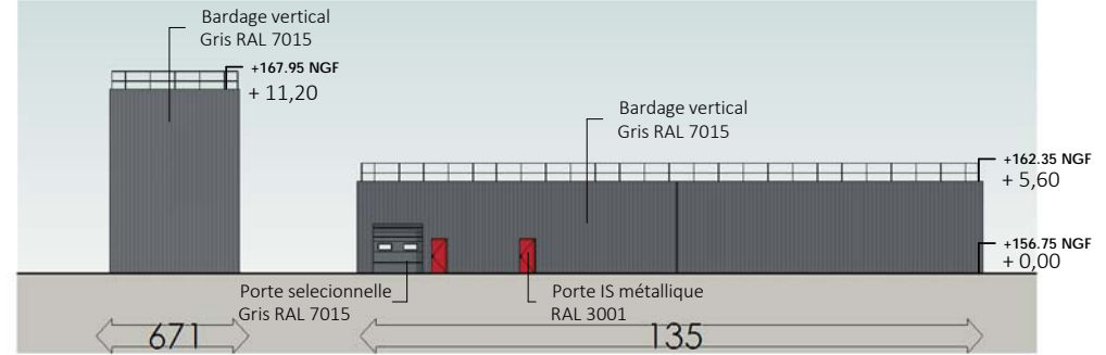
4 Façade Nord 1 : 500
