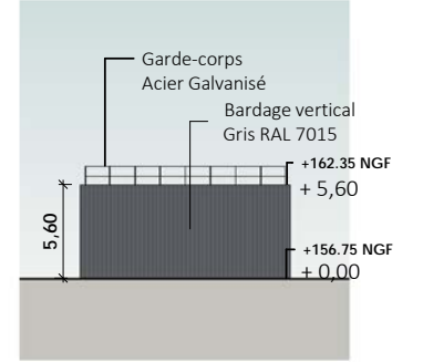
7 Façade Est -B135 1 : 500
